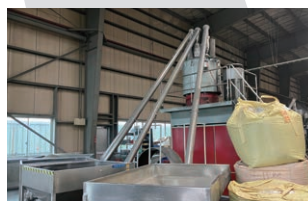
配合工程(コンパウンド加工)
